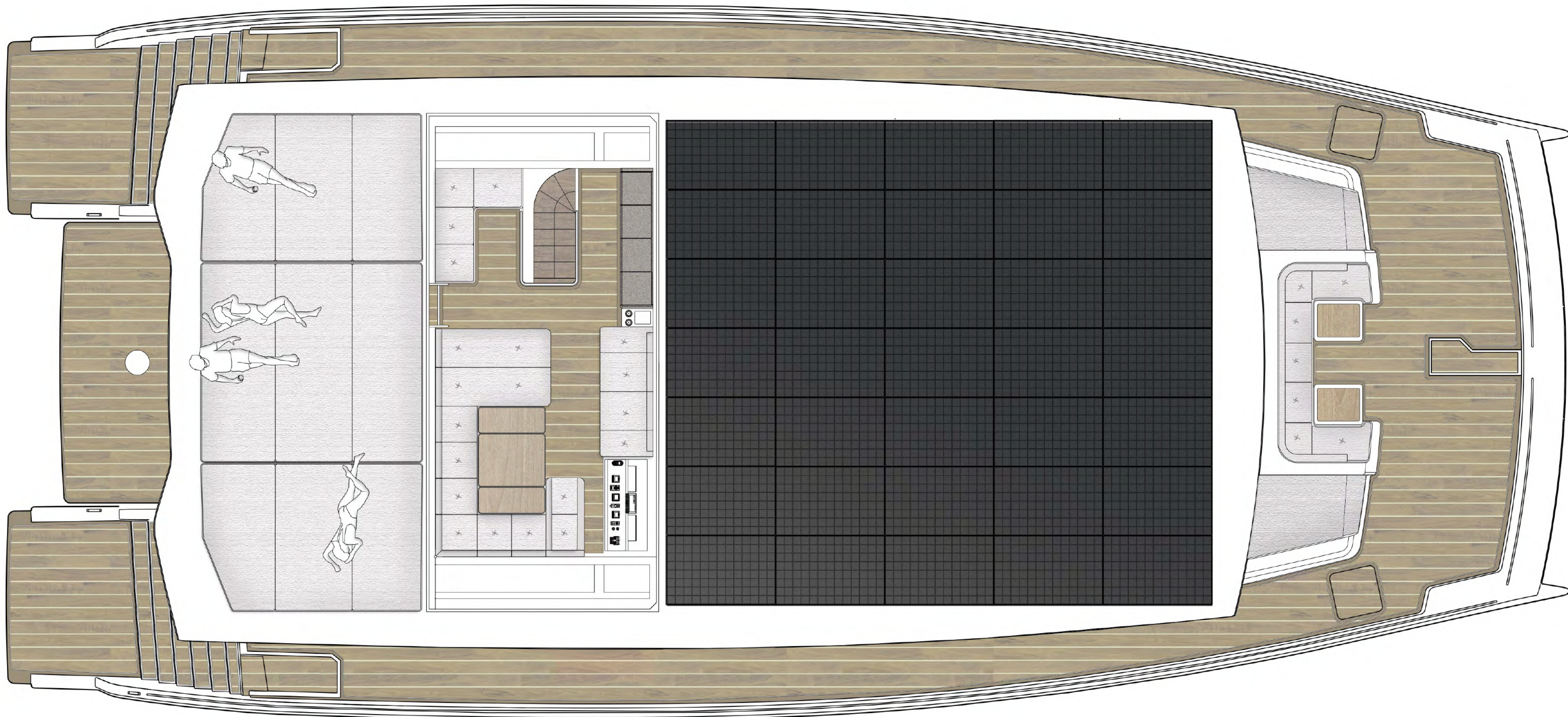
Flybridge
